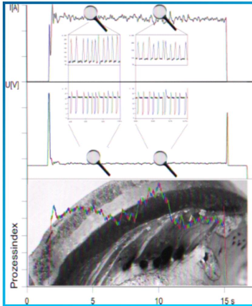
Impulzus hegesztési eljárás (varrathibák a jobboldalon)
